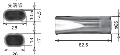
NEW β/WX 扁平ノズル 10.5・13
