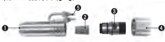
水冷ノズル 350Aセット (①~⑥)
